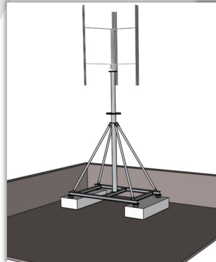
geplante Gliederung der Erneuerbaren Energieanlagen auf dem Dach des Gebäudeteils A
