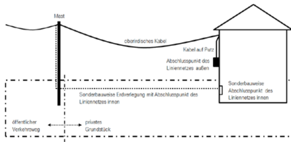
Abbildung 1 Standardbauweise bei oberirdischer Linienführung auf dem öffentlichen Verkehrsweg
