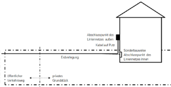
Abbildung 2 Standardbauweise bei unterirdischer Linienführung auf dem öffentlichen Verkehrsweg
